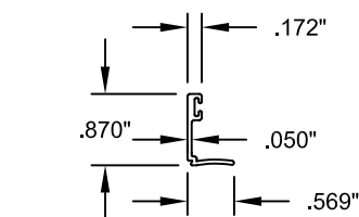
37 BEAD D #7059, 6063-T6
