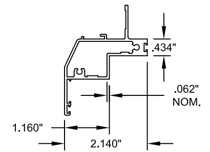
3 SASH TOP, BOTTOM & SIDE #7003, 6063-T6
