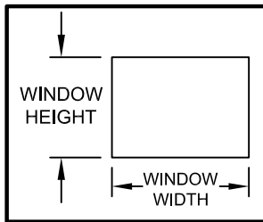
Design Pressure (psf) for Single Windows, All Anchor Groups Window Width under 23" 25-15/16" 27-7/8" 30-3/4" 32" 34" 37" 46" 53-1/8" 60" Window Height under 23" +70/-90 +70/-90 +70/-90 +70/-90 +70/-90 +70/-90 +70/-90 +70/-90 +70/-90 +70/-90 +70/-90 25-15/16" +70/-90 +70/-90 +70/-90 +70/-90 +70/-90 +70/-90 +70/-90 +70/-90 +70/-90 +70/-90 +70/-90 39" +70/-90 +70/-90 +70/-90 +70/-90 +70/-90 +70/-90 +70/-90 +70/-90 +70/-90 +70/-90 +70/-81.2 50-5/8" +70/-90 +70/-90 +70/-90 +70/-90 +70/-90 +70/-90 +70/-90 +70/-88.8 60" +70/-90 +70/-90 +70/-90 +70/-90 +70/-90 +70/-90 +70/-84.6 63" +70/-90 +70/-90 +70/-90 +70/-90 +70/-90 +70/-86.1 +70/-79.9 67" +70/-90 +70/-90 +70/-90 +70/-87 +70/-83.6 +70/-79.1 72" +70/-90 +70/-90 +70/-88.2 +70/-79 +70/-74.6 76" +70/-90 +70/-90 +70/-85.8 +70/- 74 84" +70/-90 +70/-90 +70/-80.8
