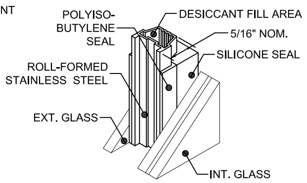
103 XL EDGE™ SPACER
