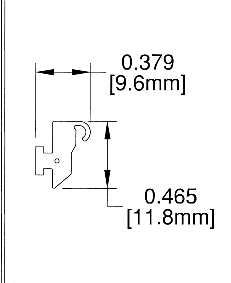
⑥ EDGE GASKET GA-25SH EPDM
