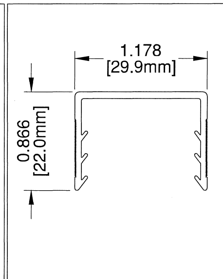
15 'U' CAP GASKET GAEP01 EPDM
