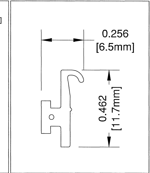
13 EDGE GASKET GA-25SH EPDM
