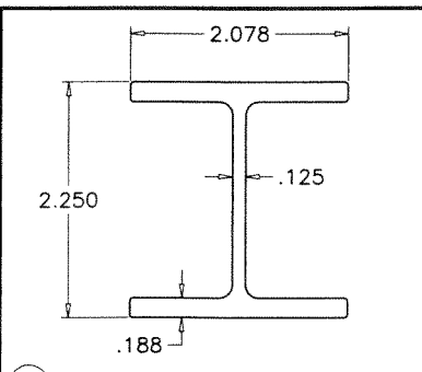
ALUM. ASTRAGAL STIFFENER
