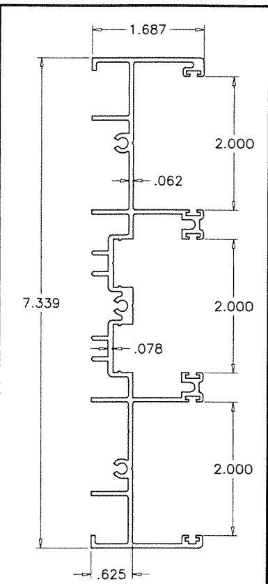
FRAME JAMB
