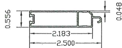
2A- BOTTOM BLADE 6063-T6 ALLOY (min. Fty= 23.1 Ksi)
