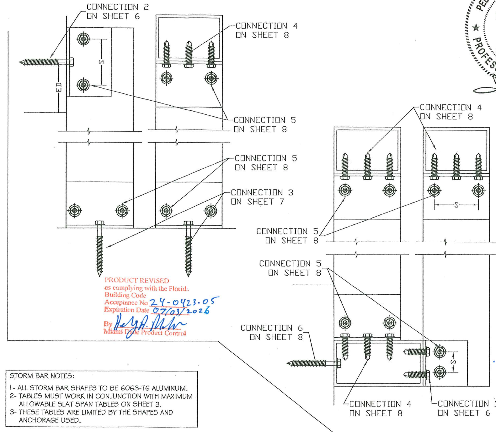
2x2 STORM BAR - 3+ SPANS
