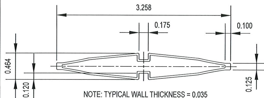
PVC SPACER SCALE 1:1
