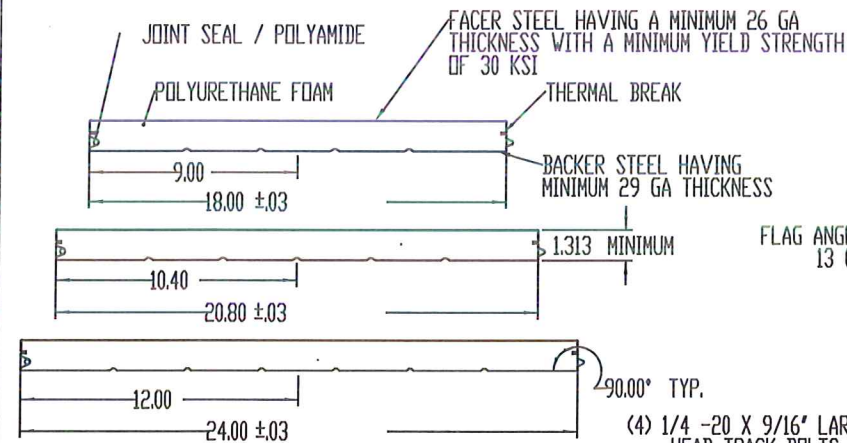
SECTION A-A SCALE 1 : 4
