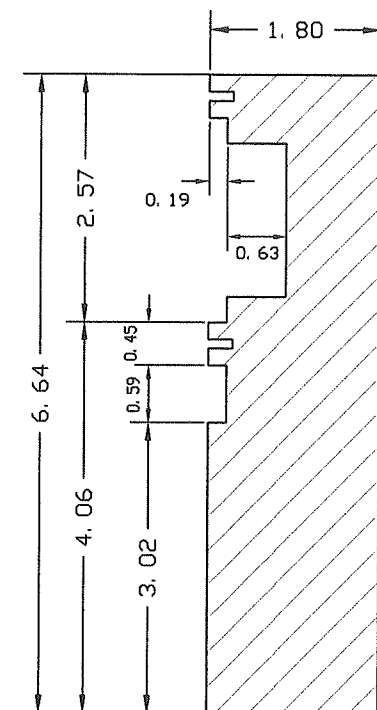
9- SIDE JAMB
