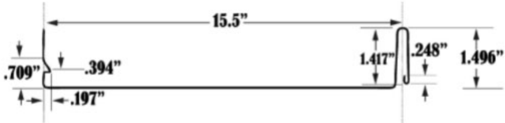
24ga. steel 1.5" SL-LOK
