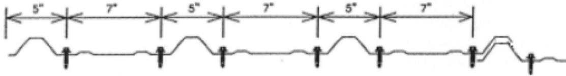
5"-7"-5"-7"-5"-7" Fastening Pattern
