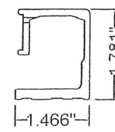
4 G-Channel 6063-T5
