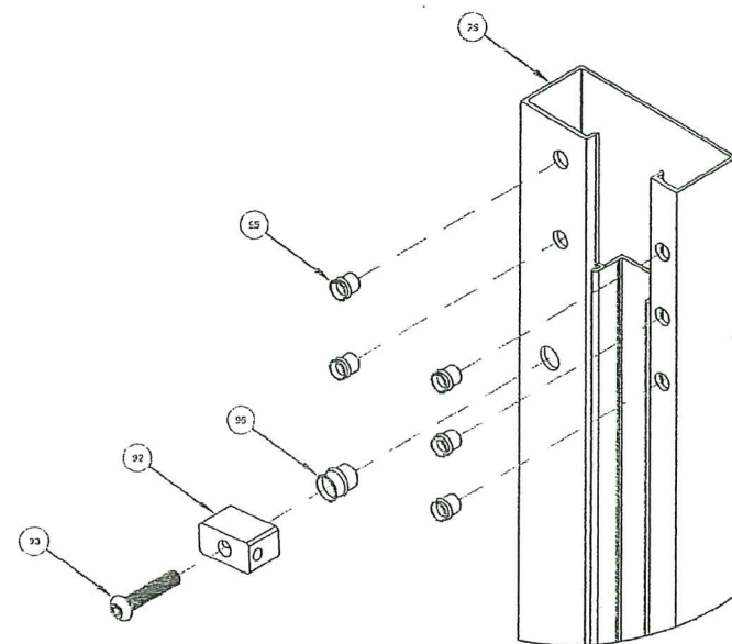
JAMB ASSEMBLY
