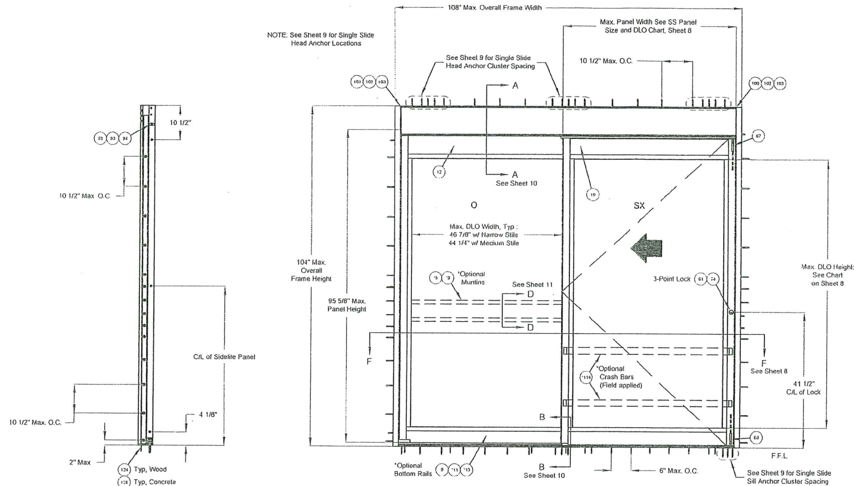
SIDELITE JAMB
