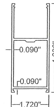
9 H4 6063-T5
