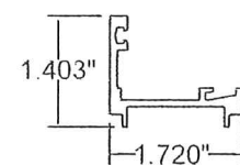
25 Gutter 6063-T5
