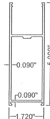
10 H5 6063-T5
