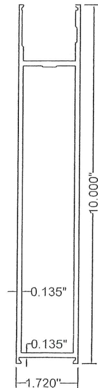
13 H10 6063-T5
