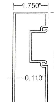
26 Jamb 6063-T6
