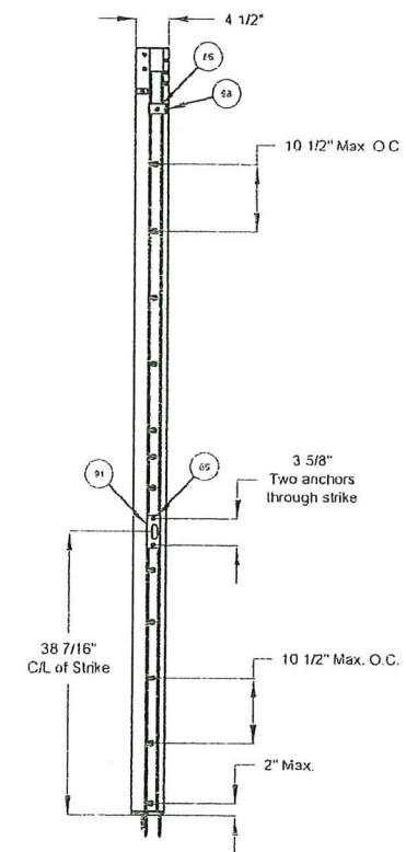
ACTIVE JAMB
