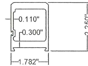
14 V2N 6063-T5
