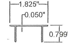
27 Jamb Snap 6063-T6
