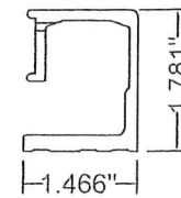
4 G-Channel 6063-T5
