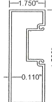
26 Jamb 6063-T6
