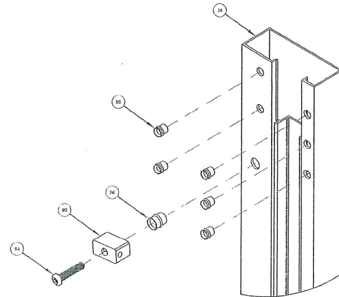
JAMB ASSEMBLY
