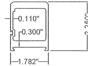
14 V2N 6063-T5
