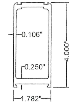
17 V1M 6063-T5
