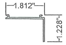
18 S/L Cap 6063-T5
