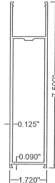
12 H7.5 6063-T6
