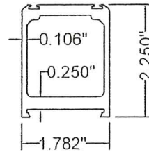
15 V1N 6063-T5
