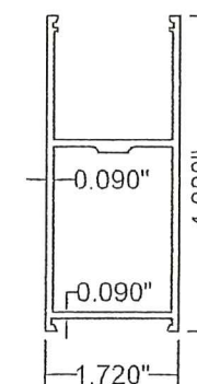
9 H4 6063-T5
