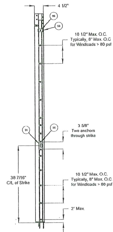
ACTIVE JAMB
