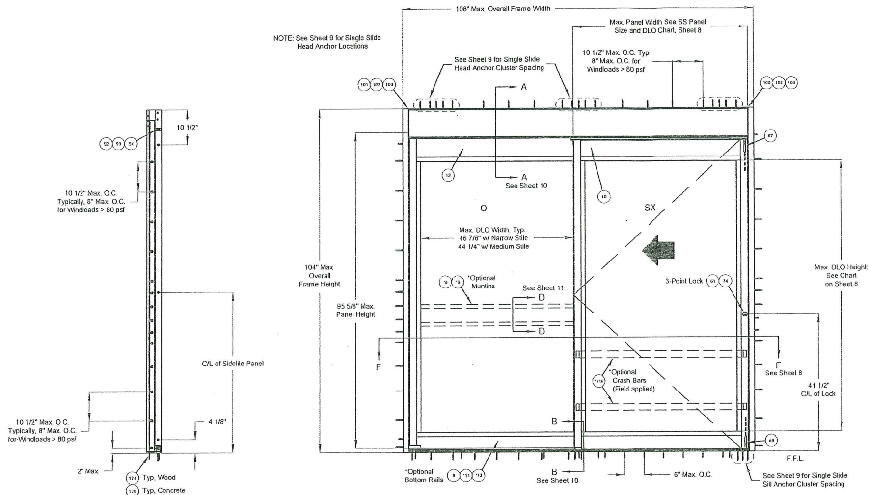
SIDELITE JAMB
