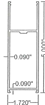
10 H5 6063-T5
