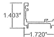
25 Gutter 6063-T5
