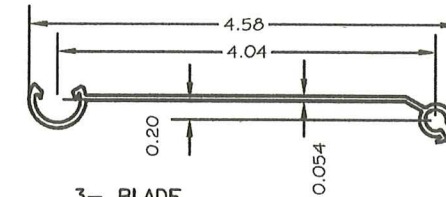
3- BLADE
