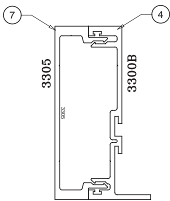
JAMB ‘J1’
