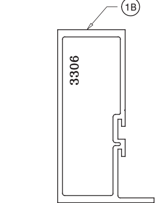
JAMB ‘J3’
