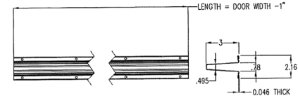
3" STRUT OPEN EN. (UBAR) 80 KSI MIN. YIELD STRENGTH, 3" X 18GA
