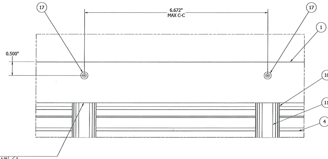
11 HEAD CONNECTION DETAILS 2,3,4 N.T.S.
