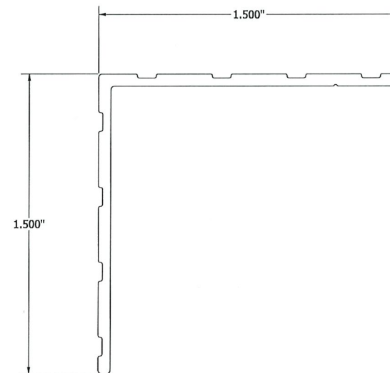
ITEM 7 CORNER LUG N.T.S. RUSKIN PART # RSM285
