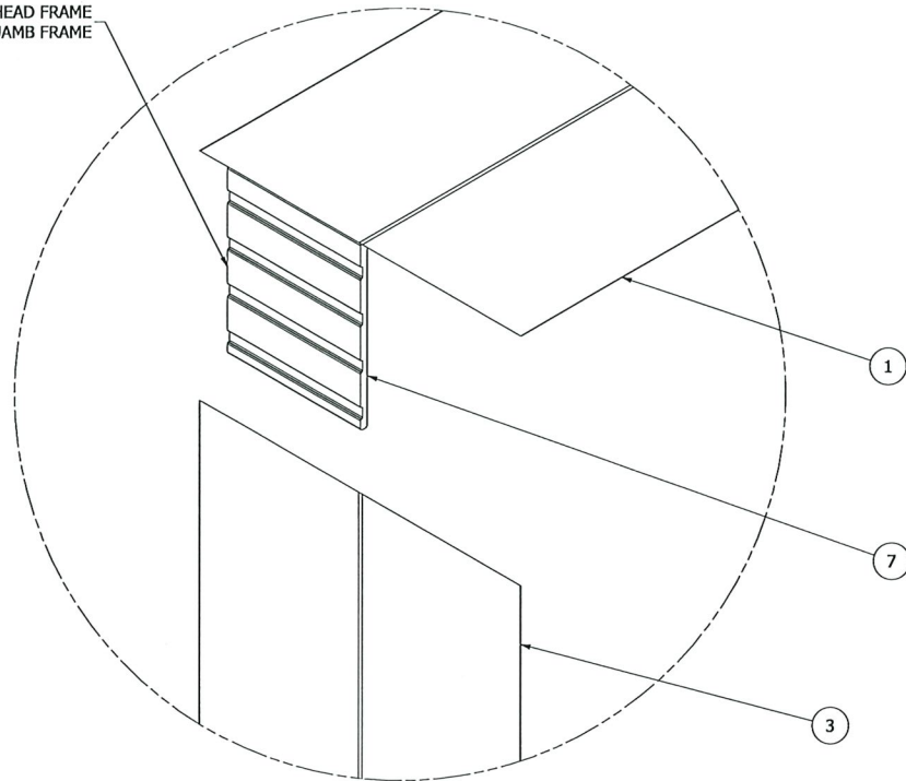
8 CORNER CONNECTION DETAILS 2,3,4 N.T.S.
