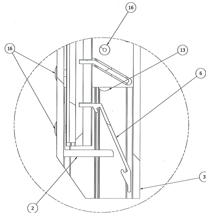
5 SILL CONSTRUCTION DETAILS 2,3,4 N.T.S.
