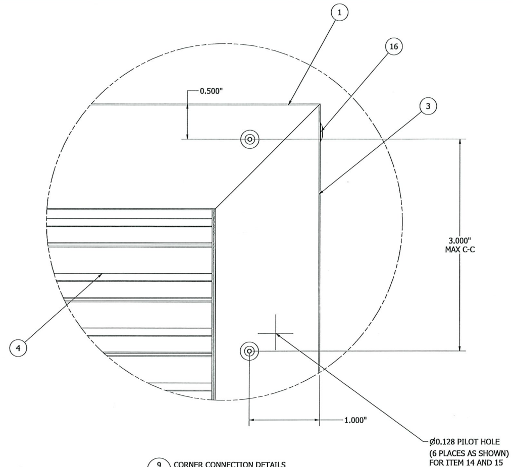
9 CORNER CONNECTION DETAILS 2,3,4 N.T.S.
