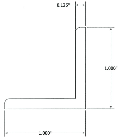
ITEM 2 SILL ANGLE N.T.S.
