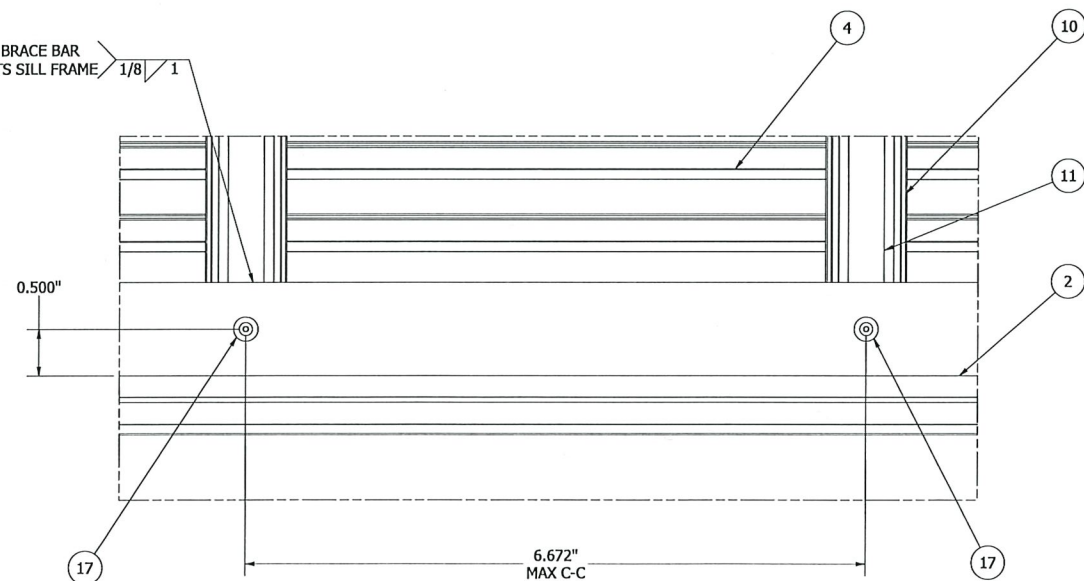
10 SILL CONNECTION DETAILS 2,3,4 N.T.S.
