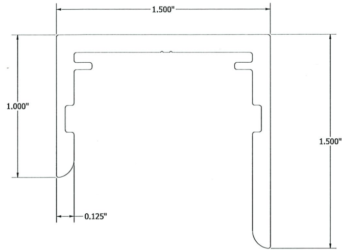
ITEM 1 & 3 HEAD & JAMB FRAME N.T.S. RUSKIN PART # 70-023371-00B
