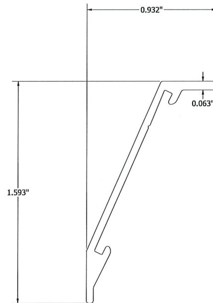
ITEM 6 BOTTOM BLADE N.T.S. RUSKIN PART # RSM68
