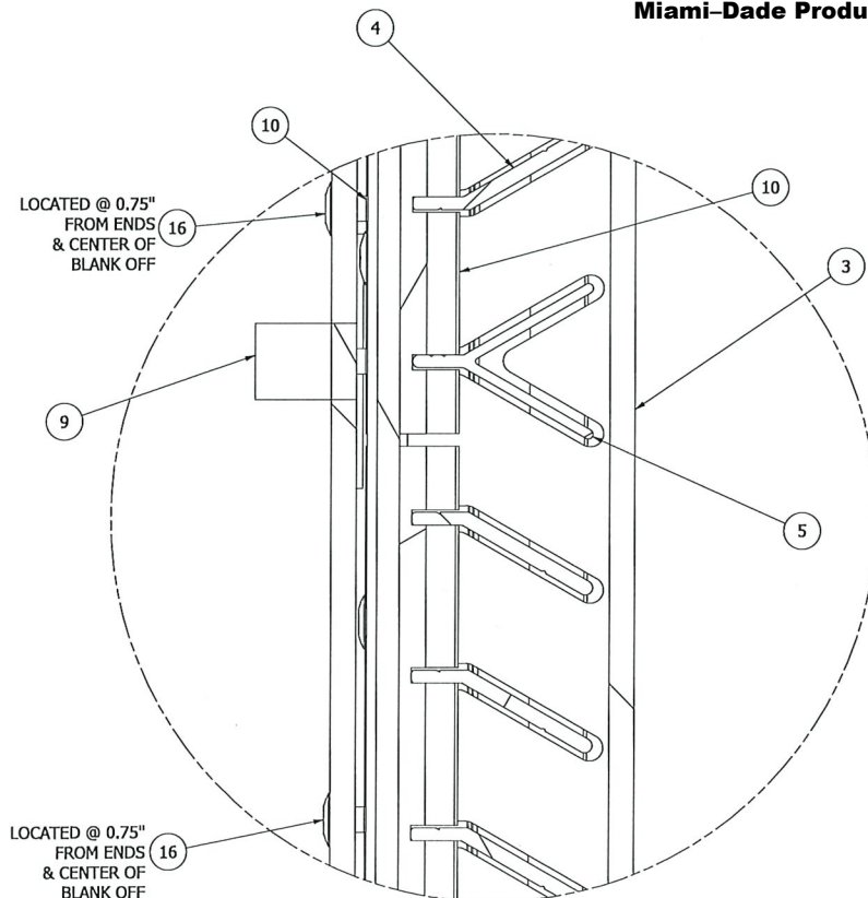
4 Y BLADE CONSTRUCTION DETAILS 2,3,4 N.T.S.
