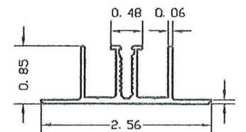
4- 3mm-4mm CENTER BASE #SAP 9014233
