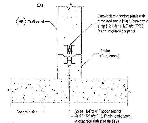
4 DETAIL 4 SCALE: 1-1/2" = 1'-0"
