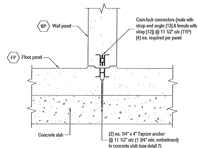
6 DETAIL 6 SCALE: 1-1/2" = 1'-0"
