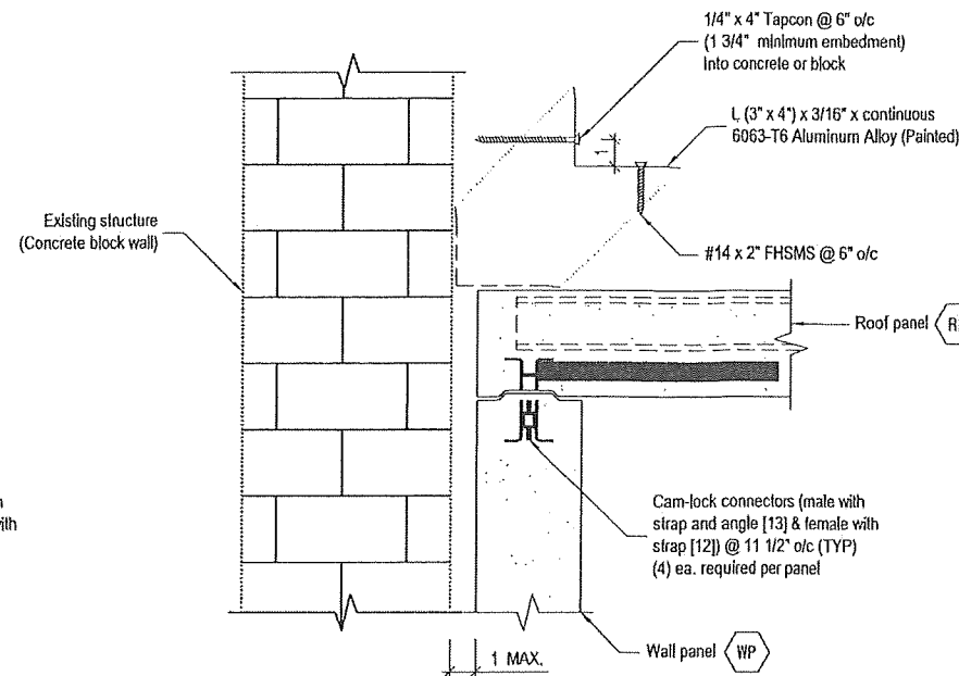
3 DETAIL 3 SCALE: 1-1/2" = 1'-0"
