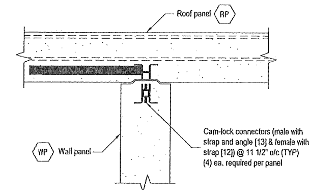
5 DETAIL 5 SCALE: 1-1/2" = 1'-0"
