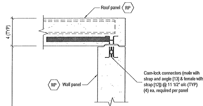
1 DETAIL 1 SCALE: 1-1/2" = 1'-0"
