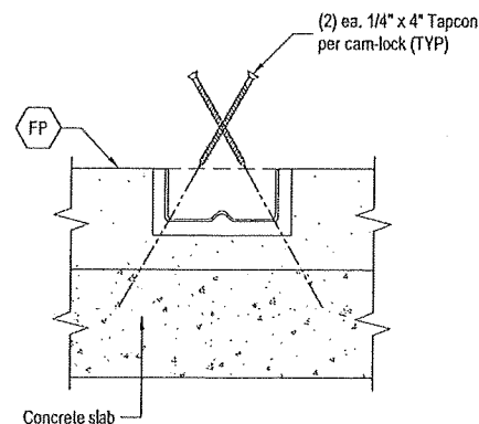
7 DETAIL 7 SCALE: 1-1/2" = 1'-0"
