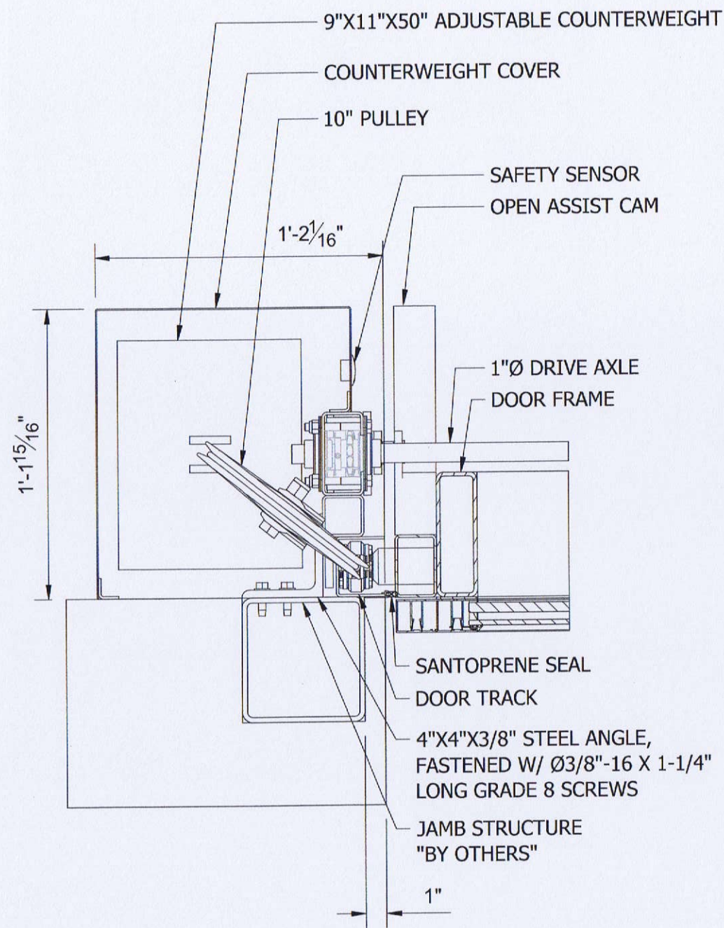
01 JAMB DETAIL
