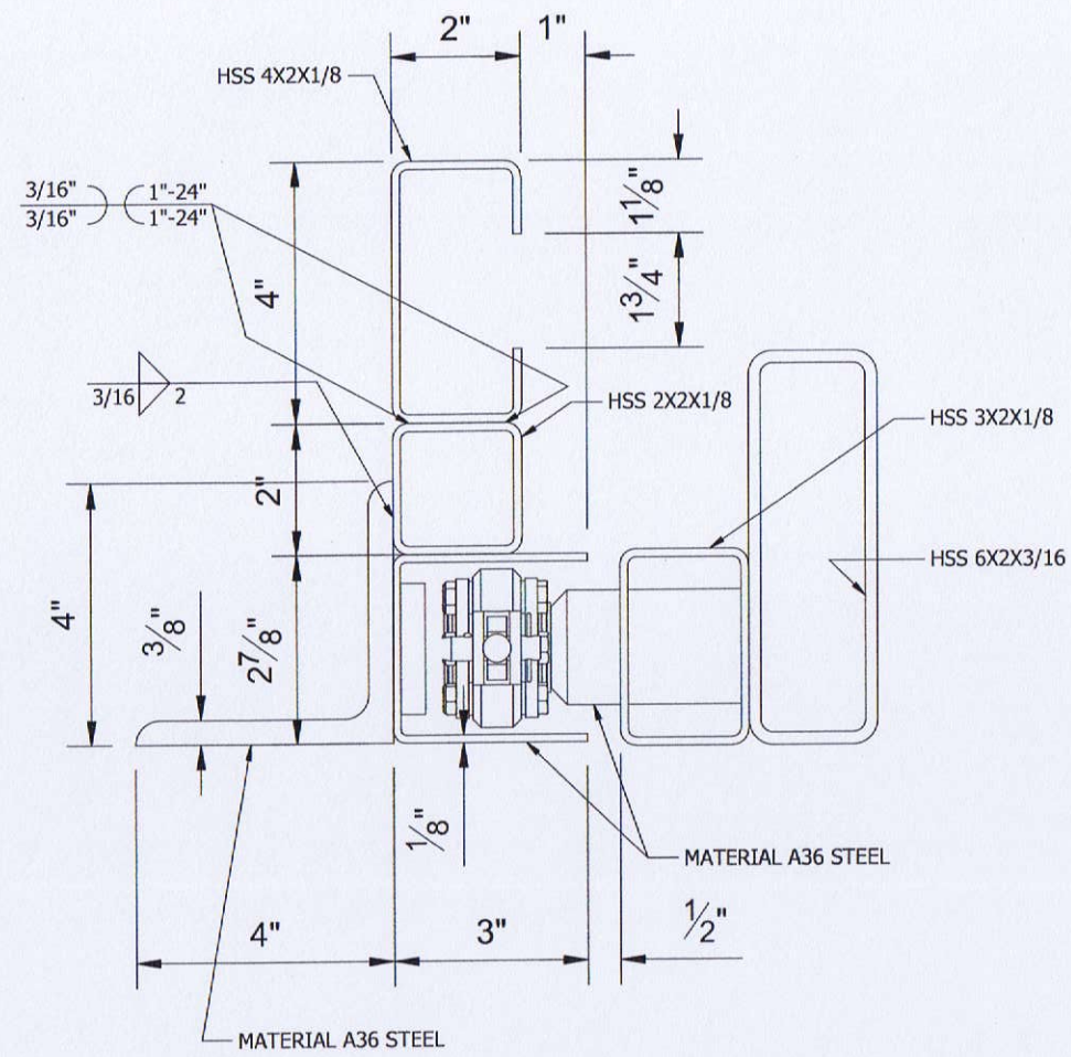
01 JAMB DETAIL TYP.
