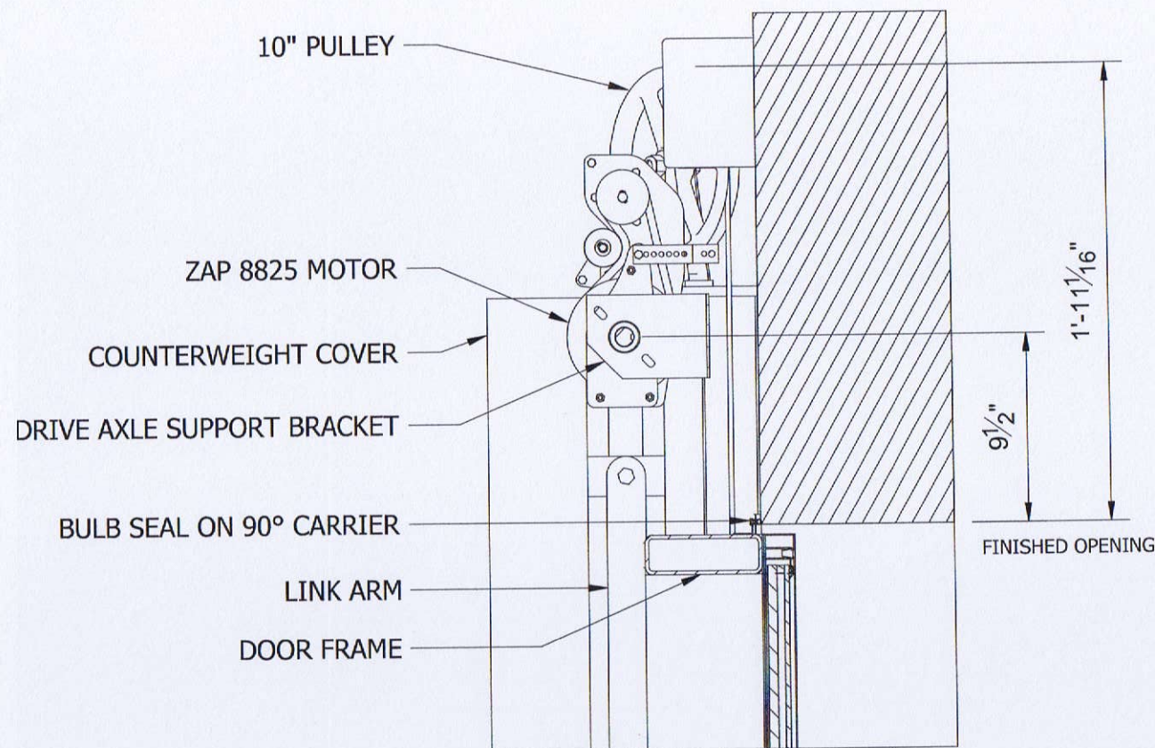
01 DOOR HEAD
