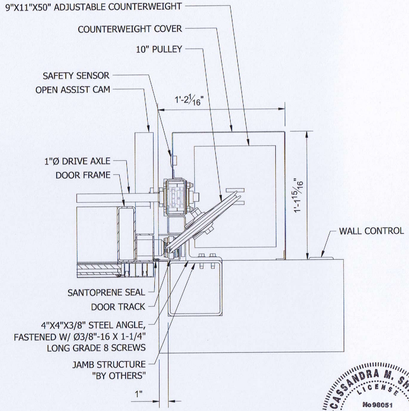
02 JAMB DETAIL
