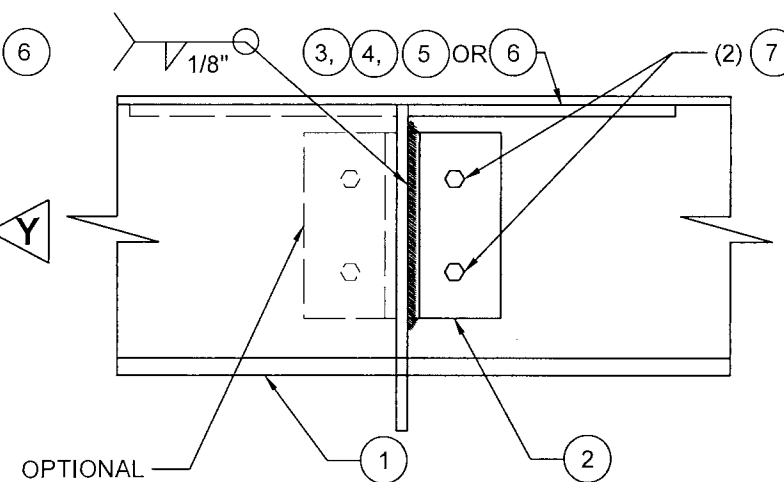
VIEW Y
