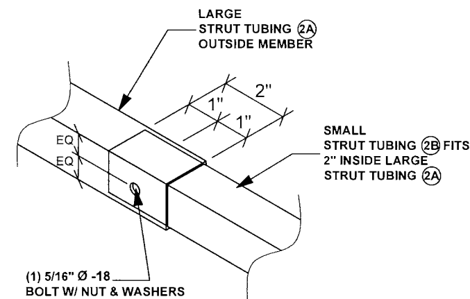
3 STRUT SPLICE SCALE: 1/4"= 0'- 1"
