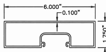
2 JAMB 6 N.T.S. 6063-T6
