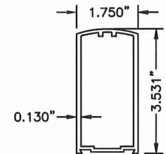
12 STILE LEAD (MEDIUM) N.T.S. 6063-T6
