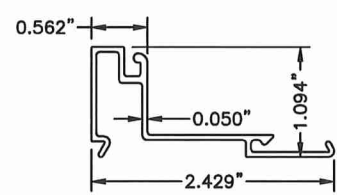
89 TRANSOM IG GUTTER N.T.S. 6063-T6 HEADER
