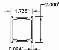
17 MUNTIN BAR N.T.S. 6063-T6
