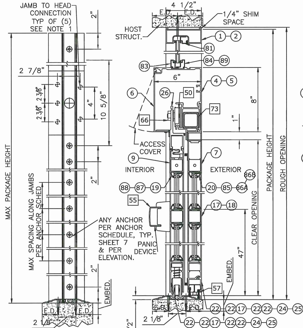
FRAME ANCHORING N.T.S.
