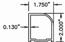
13 STILE PIVOT (NARROW) N.T.S. 6063-T6
