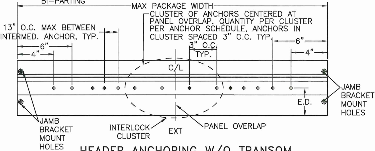
HEADER ANCHORING W/O TRANSOM N.T.S.
