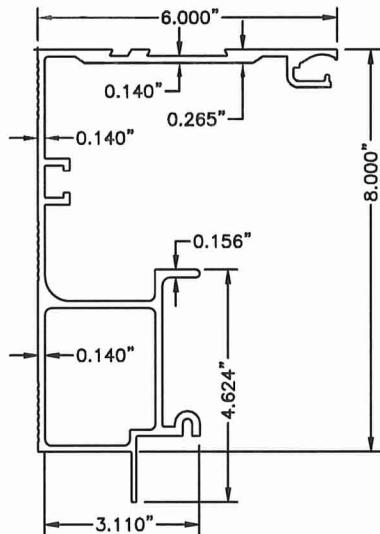
4 HEADER N.T.S. 6063-T6
