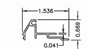
20 1/4" GUTTER N.T.S. 6063-T6 HORIZONTAL
