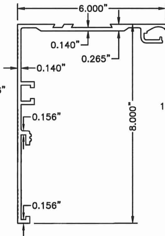
5 HEADER (2 PC.) N.T.S. 6063-T6
