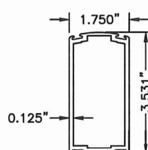
16 STILE LOCK (MEDIUM) N.T.S. 6063-T6
