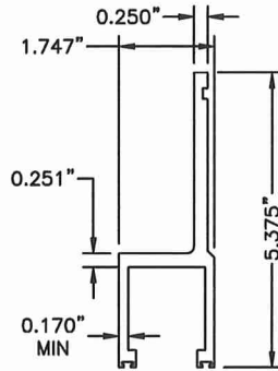
26 HANGER N.T.S. 6063-T6
