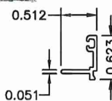
88 IG STOP N.T.S. 6063-T6
