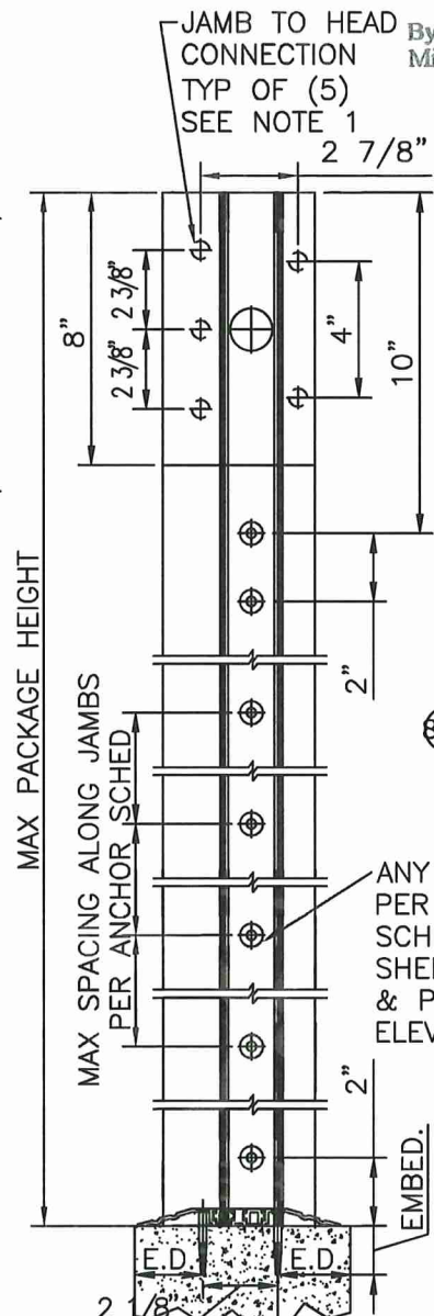
FRAME ANCHORING N.T.S.
