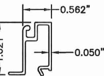
82 TRANSOM VERT. N.T.S. 6063-T6
