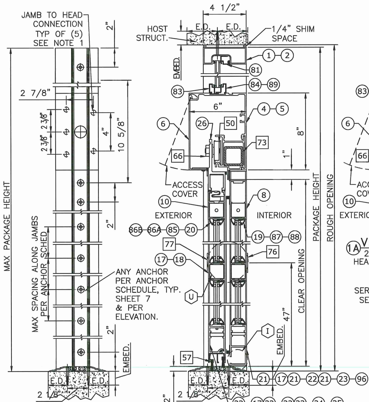
FRAME ANCHORING N.T.S.
