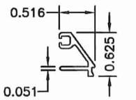
19 1/4" STOP N.T.S. 6063-T6 HORIZONTAL
