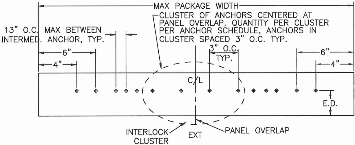
HEADER ANCHORING WITH TRANSOM N.T.S.
