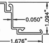
84 TRANSOM 1/4" GUTTER N.T.S. 6063-T6 HEADER
