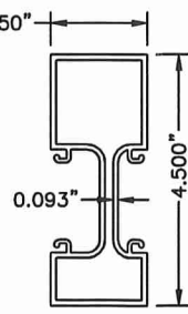
80 TRANSOM VERT. N.T.S. 6063-T6
