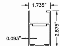
9 TOP RAIL, SX N.T.S. 3000 6063-T6
