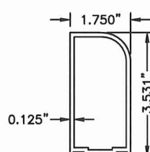
14 STILE PIVOT (MEDIUM) N.T.S. 6063-T6
