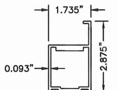
10 TOP RAIL, SX N.T.S. 2000 6063-T6
