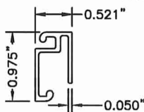
82 TRANSOM VERT. N.T.S. 6063-T6
