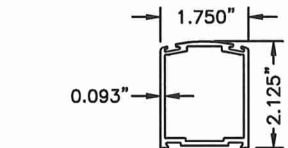
15 STILE LEAD (NARROW) N.T.S. 6063-T6
