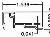
85 1/4" GUTTER N.T.S. 6063-T6 VERTICAL
