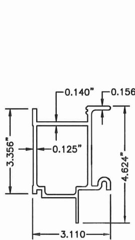
5 HEADER (2 PC.) N.T.S. 6063-T6
