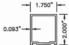
11 STILE FIXED (NARROW) N.T.S. 6063-T6
