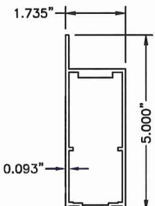
7 TOP RAIL, SO N.T.S. 3000 6063-T6
