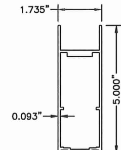
8 TOP RAIL, O N.T.S. 2000 6063-T6
