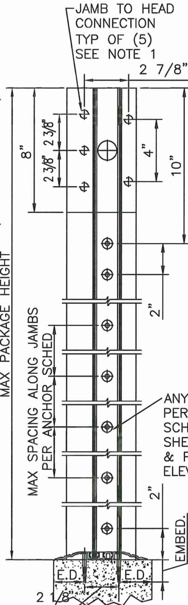
FRAME ANCHORING N.T.S.
