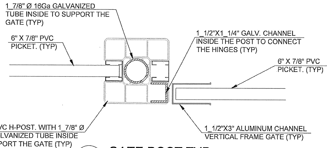
7 GATE POST TYP
