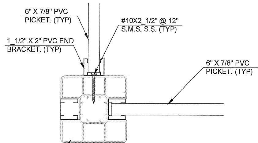
6 CORNER POST TYP
