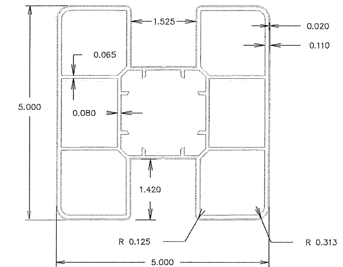
5"X5" PVC POST
