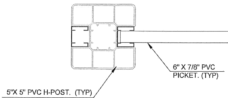
4 END POST TYP
