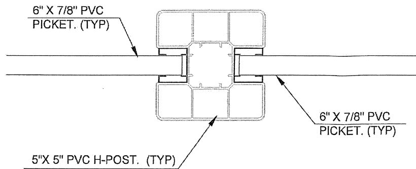
5 INTERIOR POST TYP
