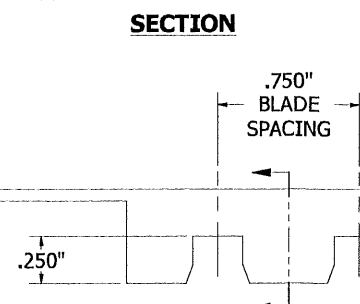
H.H.B.S. ITEM-5 N.T.S.
