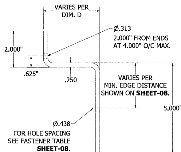
RETAINING ZEE ITEM - 15 N.T.S.
