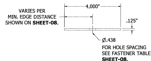
STIFFENER PLATE ITEM-19 N.T.S.
