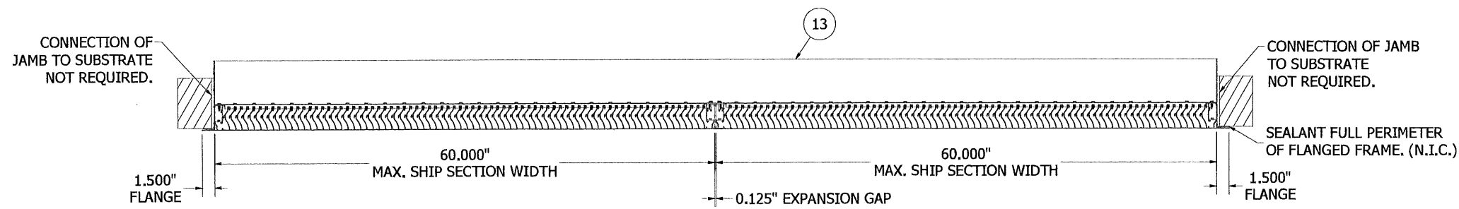
SECTION D-D
