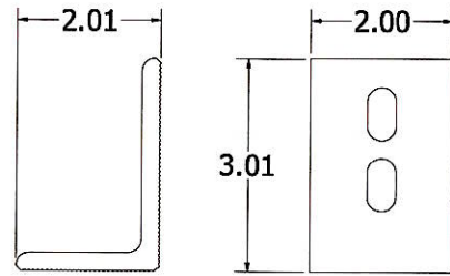
L-FOOT ITEM# 3
