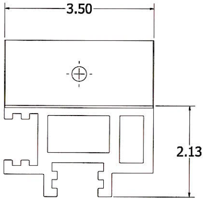
TR RISER ITEM# 3
