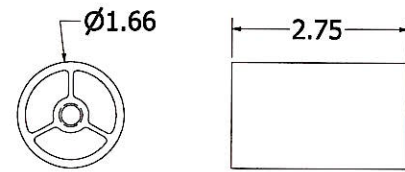
STANDOFF ITEM# 2
