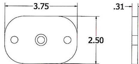
BASE ITEM# 1
