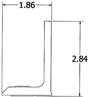
L-FOOT ITEM #2
