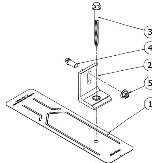
FLASHKIT PRO SB L-FOOT ORIENT 1
