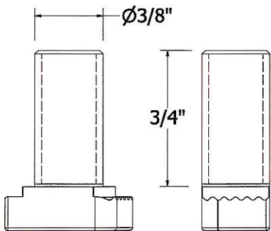
ITEM 4 3/8-16 ENHNCD T-BOLT
