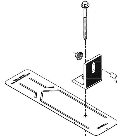
FLASHKIT PRO SB L-FOOT ORIENT 2
