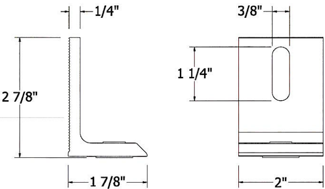
ITEM 2 L-FOOT GROMMET ASSEMBLY
