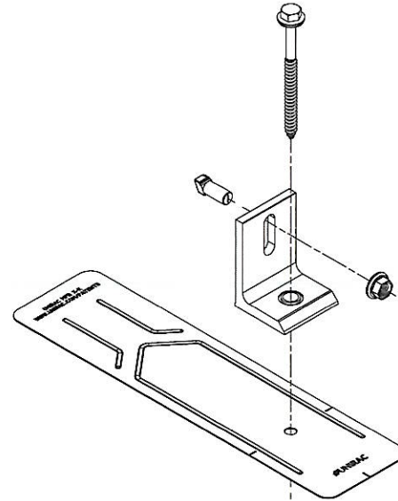
FLASHKIT PRO SB L-FOOT ORIENT 1
