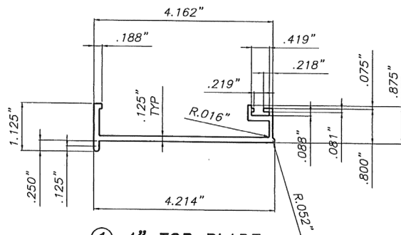
① 4" TOP BLADE SCALE: 3/8"=1"
