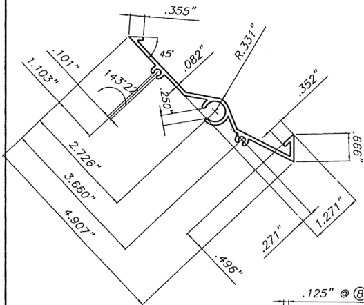
② 4" BLADE SCALE: 3/8"=1"
