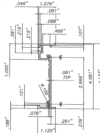
⑤ 4" SIDE JAMB SCALE: 3/8"=1"
