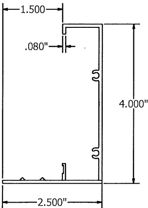
FLANGED JAMB FRAME ITEM-18 N.T.S.
