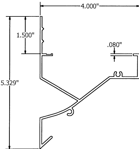
FLANGED HEAD FRAME ITEM-16 N.T.S.
