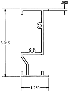
JAMB FRAME ITEM-3 N.T.S.
