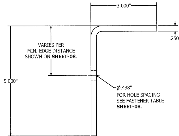
RETAINING ANGLE ITEM-26 N.T.S.
