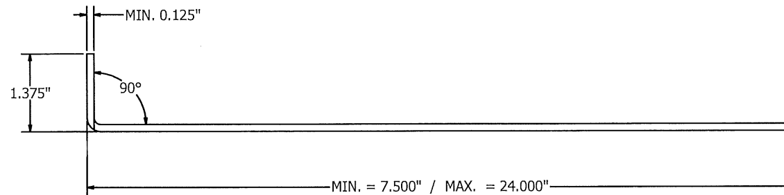
UNIVERSAL SLEEVE ITEM-22 N.T.S.
