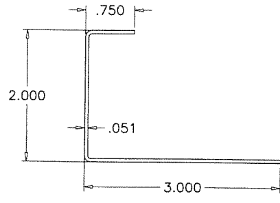
END STILE 18 GA. STEEL
