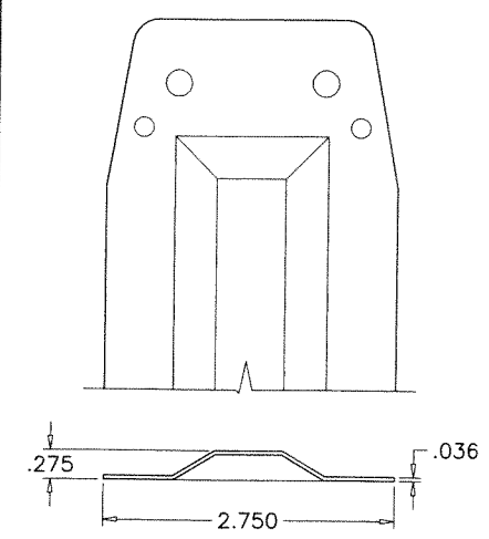
CENTER STILE 20 GA. STEEL
