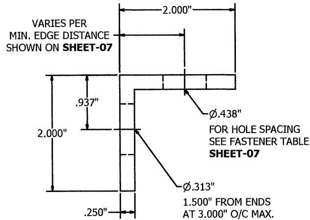
RETAINING ANGLE ITEM-19 N.T.S.
