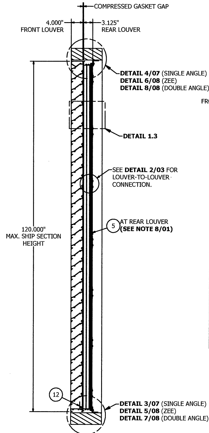
SECTION A-A
