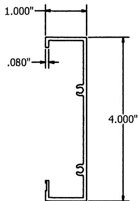
JAMB FRAME ITEM-10 N.T.S.
