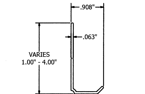
WATERSTOP ITEM-12 N.T.S.
