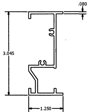
JAMB FRAME ITEM-3 N.T.S.
