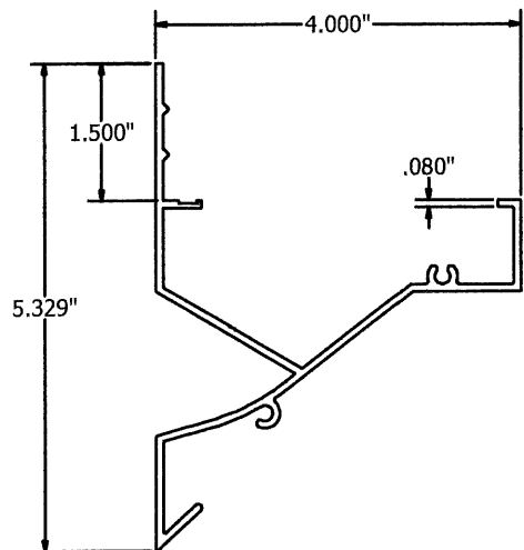
FLANGED HEAD FRAME ITEM-16 N.T.S.
