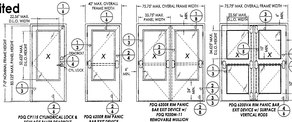
7'-0" DOOR
