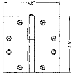
9 STEEL HINGE 0.134\"/>
