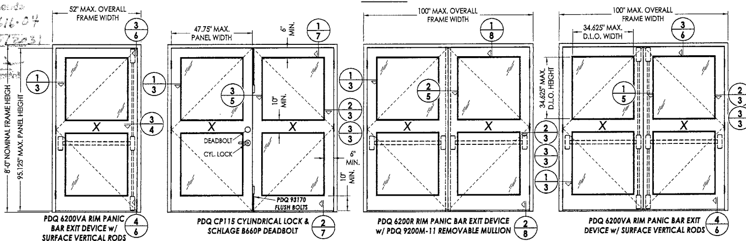
8'-0" DOOR
