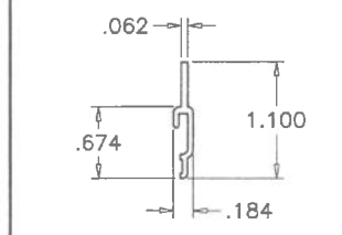
⑬ SILL RISER
