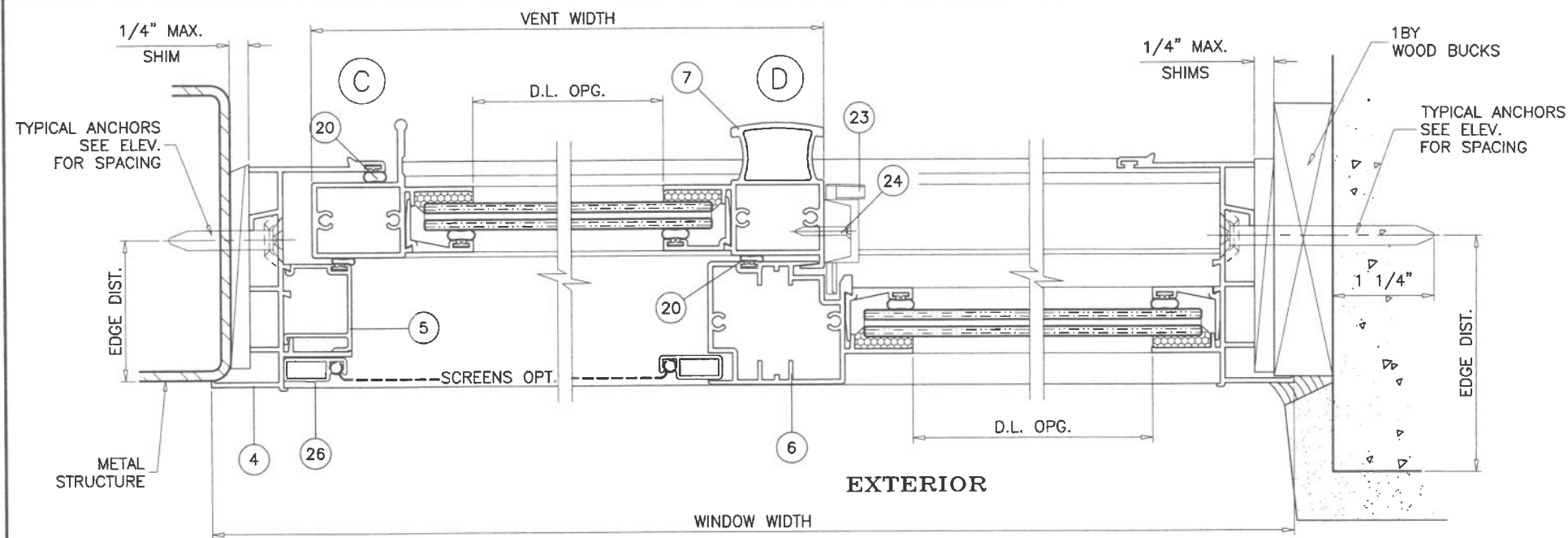
XO LAYOUT
