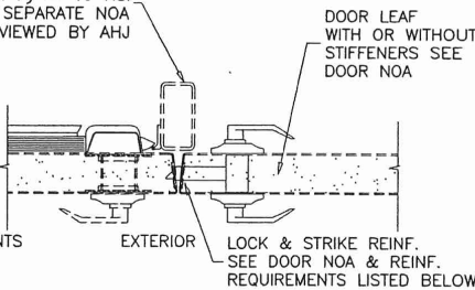
SECTION D-D
