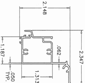
E6 VENT BOTTOM RAIL
