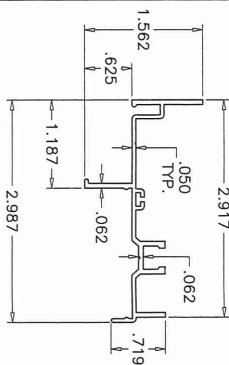
E1 FRAME HEAD
