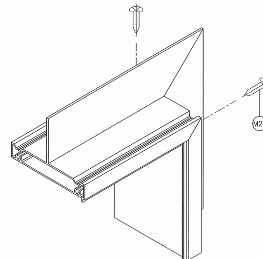
FIN FRAME ADAPTER CORNER
