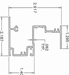
E15 FLUSH FRAME ADAPTER WITH FIN
