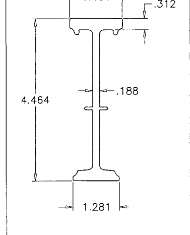
E06 STIFFENER
