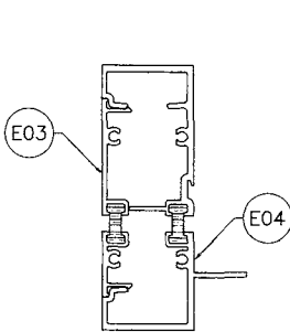
JAMB 'J1'
