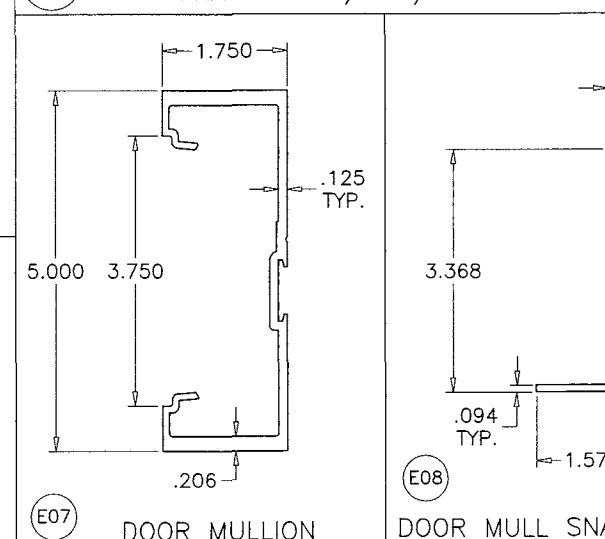
E07 DOOR MULLION
