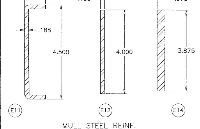
E11 E12 E14 MULL STEEL REINF.
