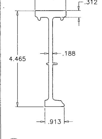
E06A STIFFENER
