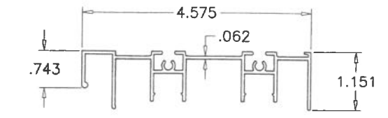
E1 FRAME HEAD
