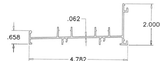
E2 FRAME SILL
