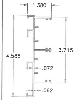
E3 FRAME JAMB
