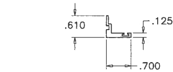
ASTRAGAL
