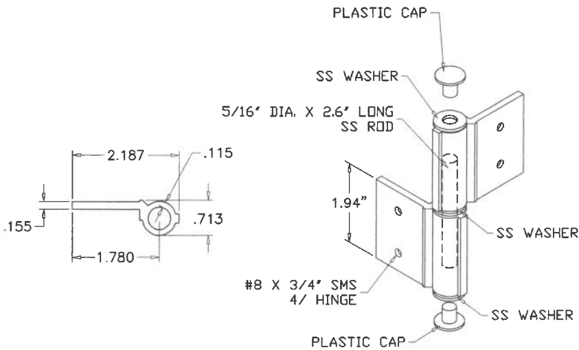
HINGE
