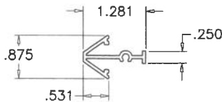
HORIZ. MUNTIN
