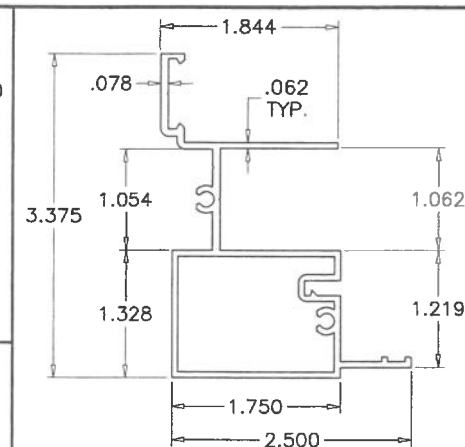
5 FRAME JAMB
