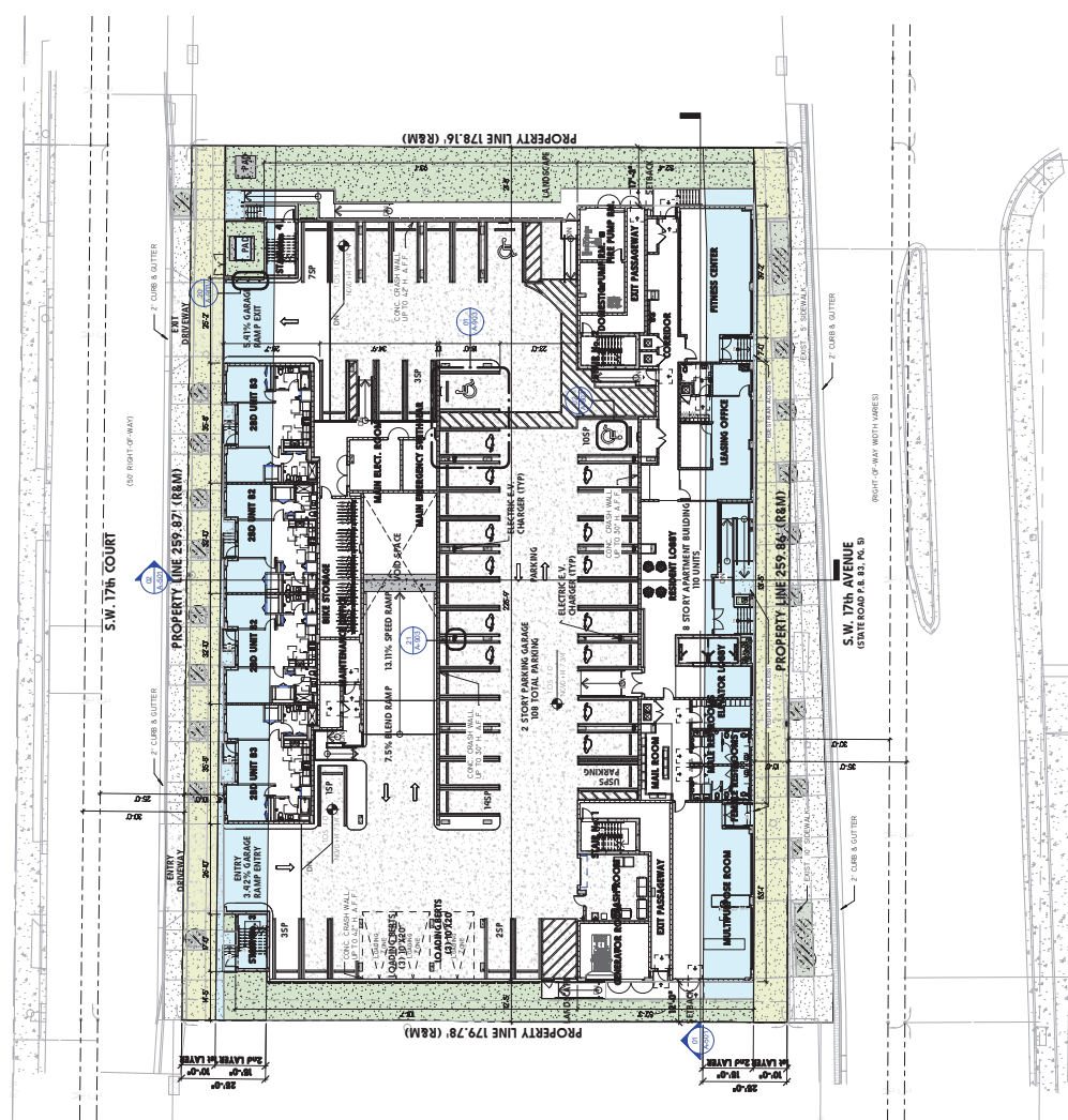
01 Site Plan SCALE: 1/8" = 1'-0"
