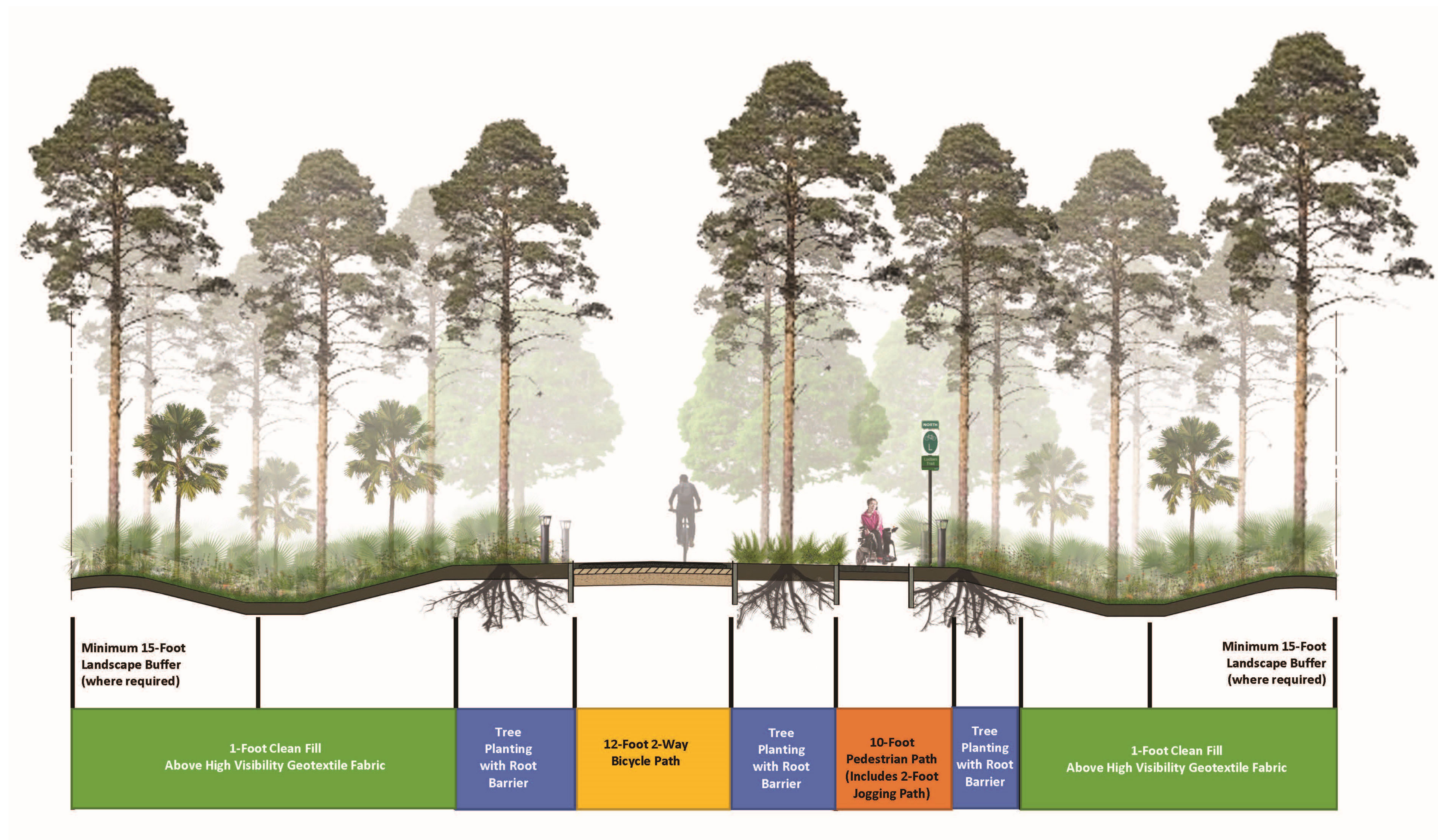
TYPICAL SECTION 1 SECCIÓN TÍPICA 1 SEKSYON TIPIK 1
