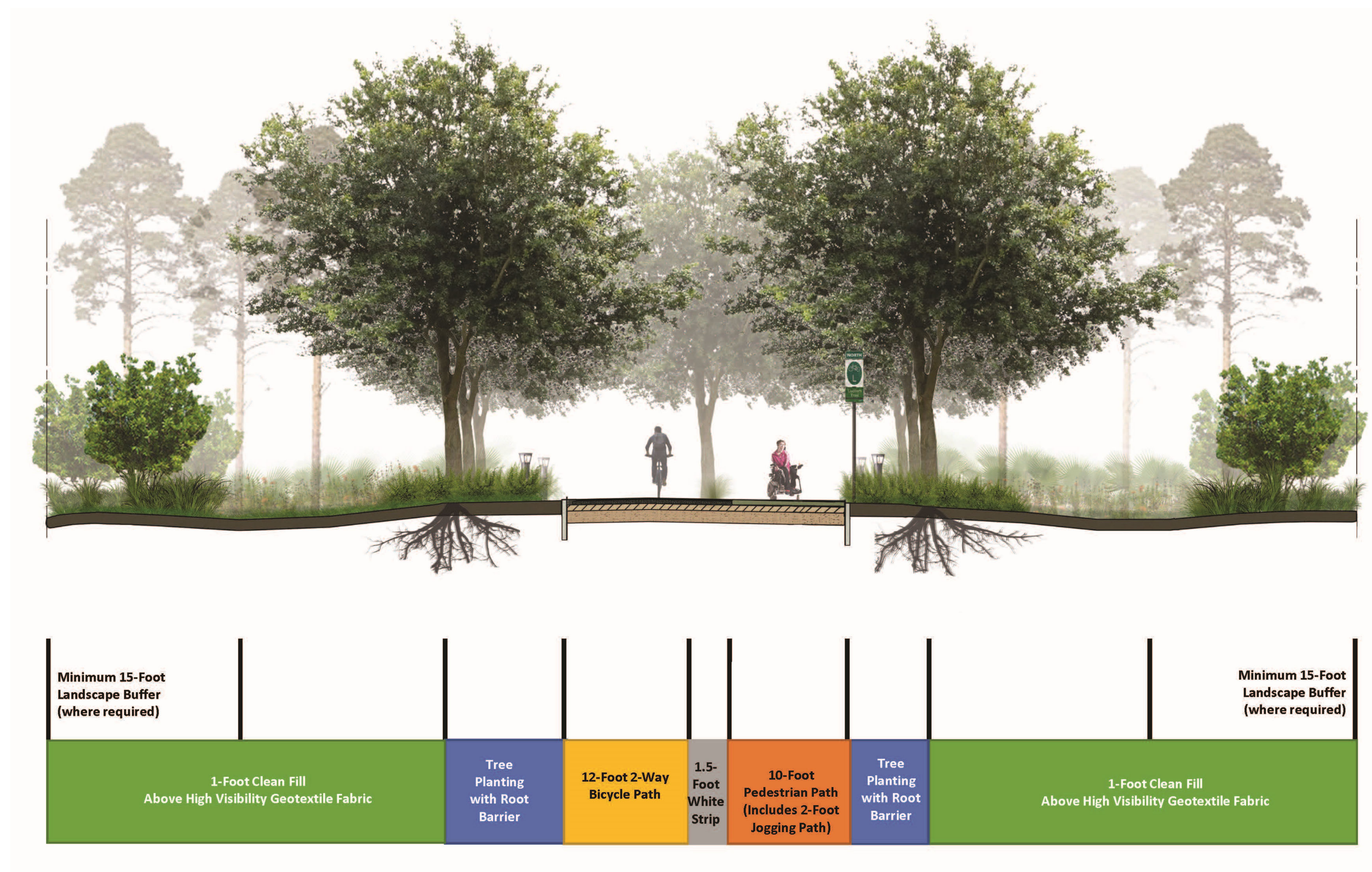
TYPICAL SECTION 2 SECCIÓN TÍPICA 2 SEKSYON TIPIK 2
